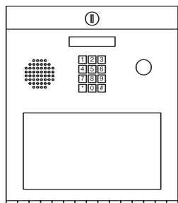
1810 Surface 11.25" W x 13" H x 4.75" D 28.5cm W x 33cm H x 12cm D
